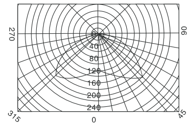
配光曲线 Cd/1000lm
