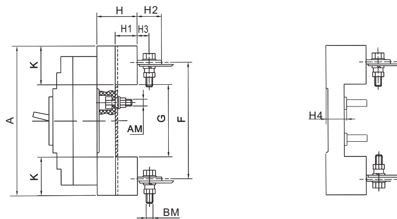
RDM7L系列插入式板后外形尺寸及安装板开孔尺寸图
