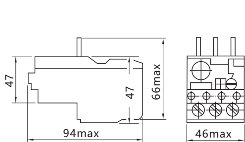
图3 RDR5-25/Z外形安装尺寸
