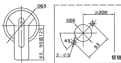
圆形延伸旋转手柄开孔尺寸图
