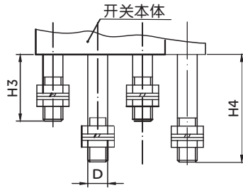
RDM5L-125、250板后接线
