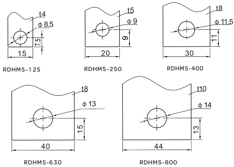
RDHM5系列推荐预制铜排尺寸
