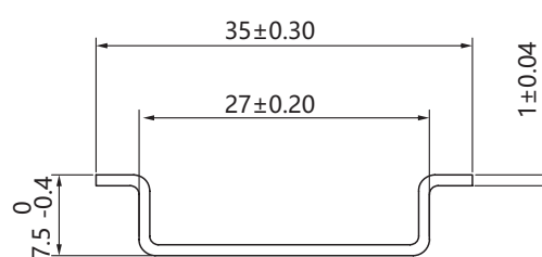
图5 安装轨尺寸
