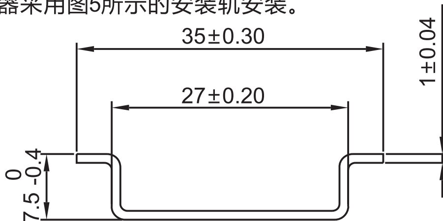
图5 安装轨尺寸
