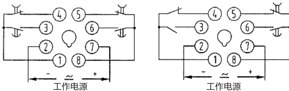
RDS3-2P RDS3-3P RDS3-2D RDS3-3D (延时2转换)
